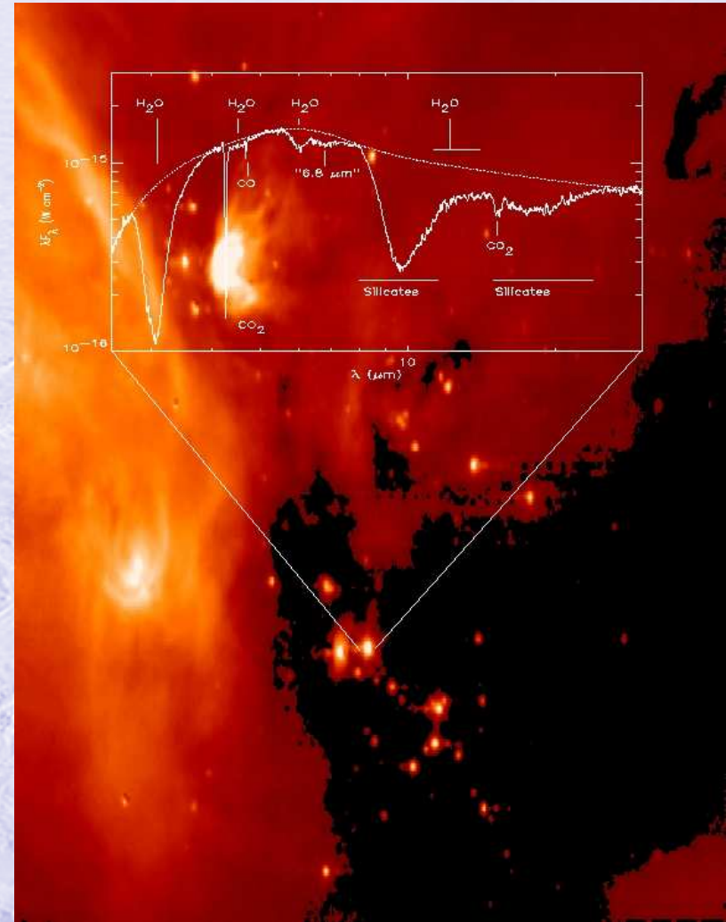
Protoestrella Elías 29 en \rho Ophiuci (500 años luz)
